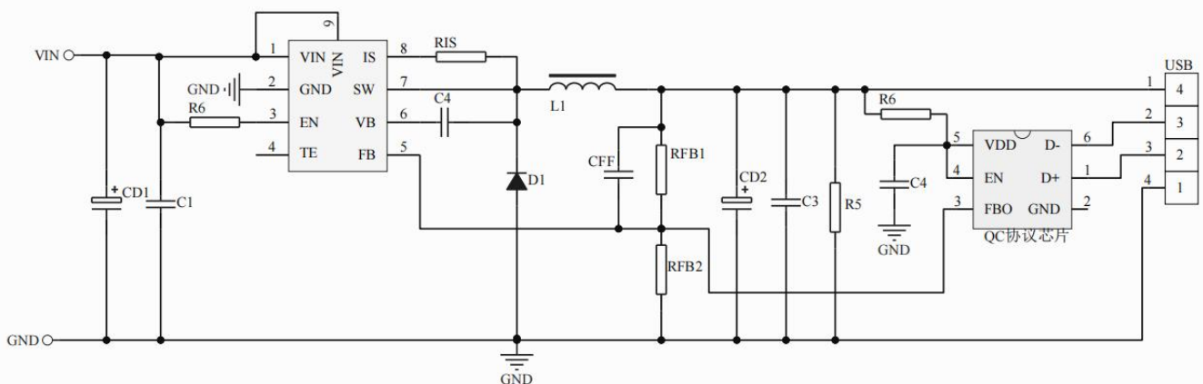
APP3: QC2.0/QC3.0
